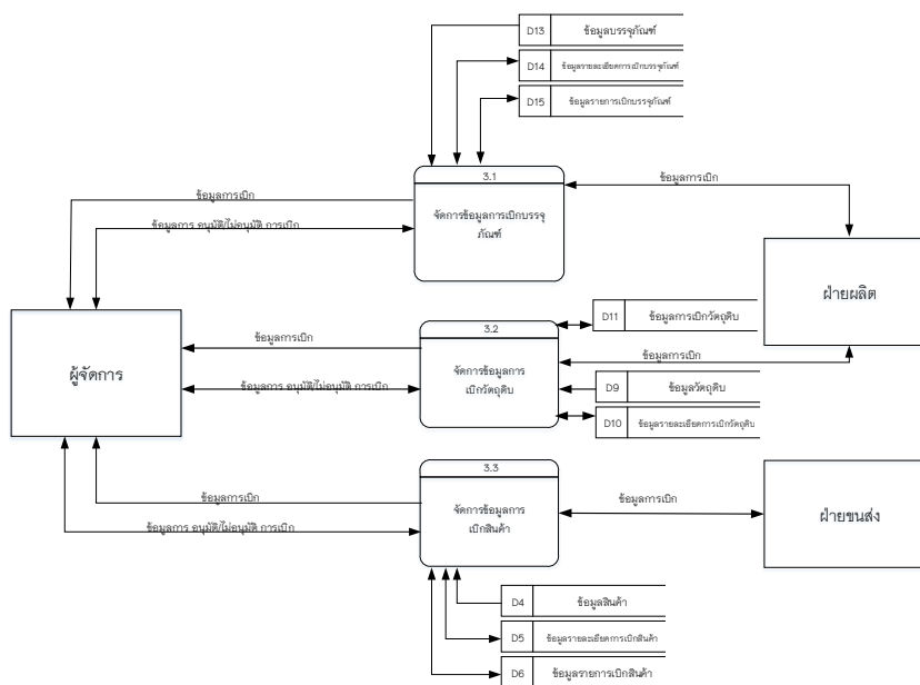
ภาพที่ 3.11 แผนภาพกระแสข้อมูลระดับที่ 1.0 จัดการข้อมูลการเบิก
