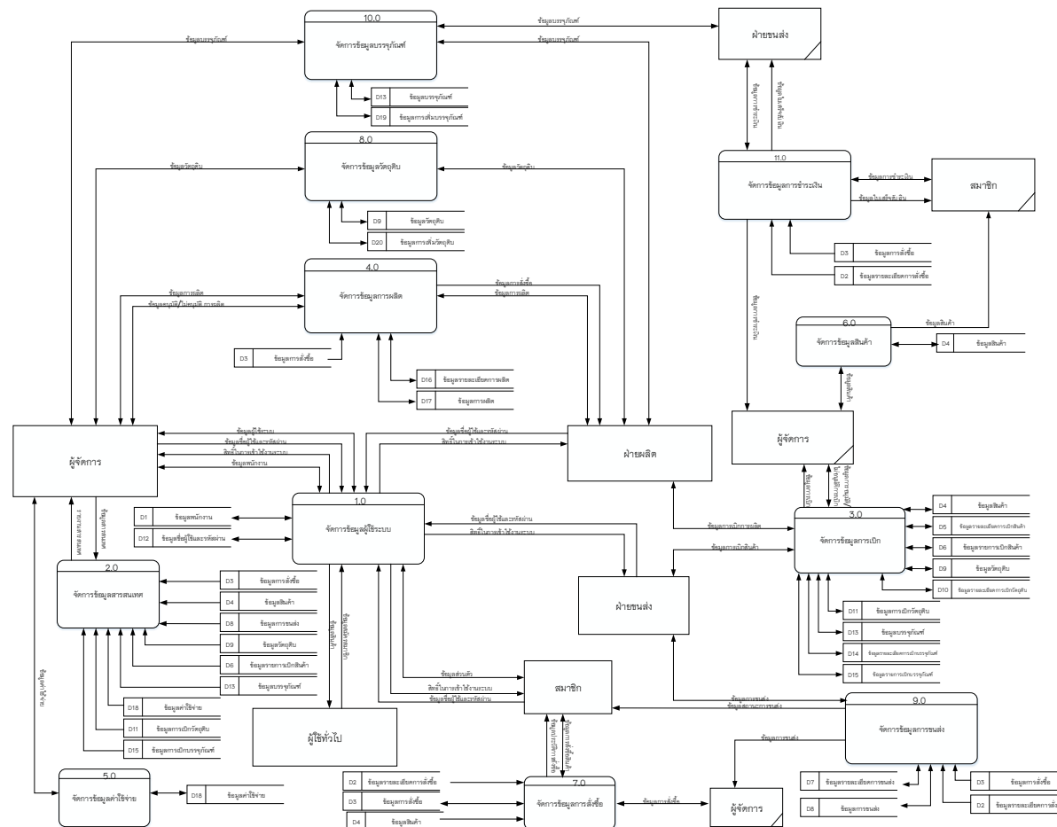
ภาพที่ 3.10 แผนภาพกระแสข้อมูลระดับที่ 0
