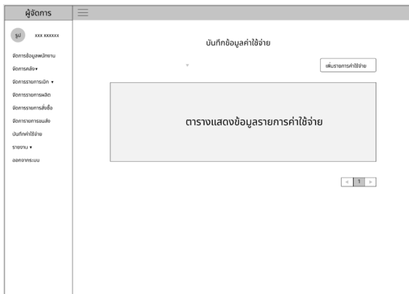
ภาพที่ 3.55 หน้าจอบันทึกข้อมูลค่าใช้จ่าย
