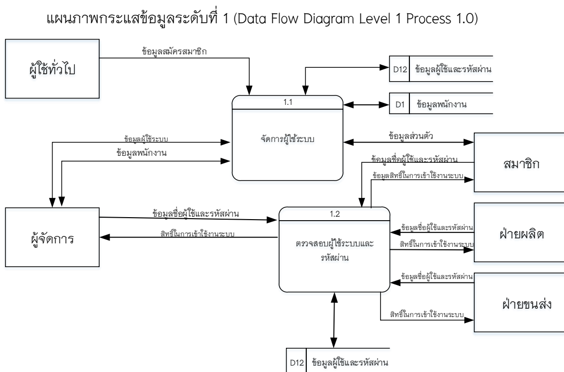
ภาพที่ 3.10 แผนภาพกระแสข้อมูลระดับที่ 1.0 จัดการข้อมูลผู้ใช้ระบบ
